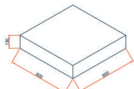
Plano alto
