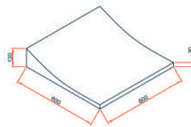
Elevação côncava
