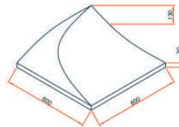
Transição LE
